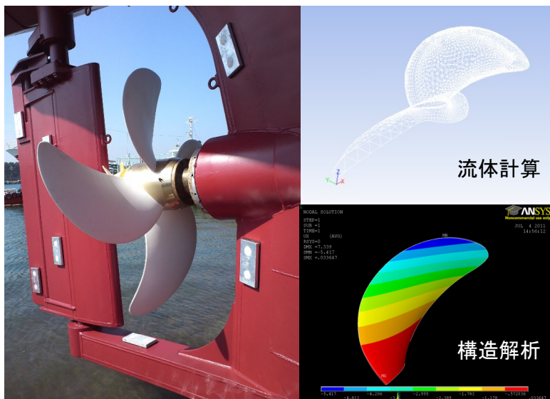
世界初の商用船CFRPプロペラ
